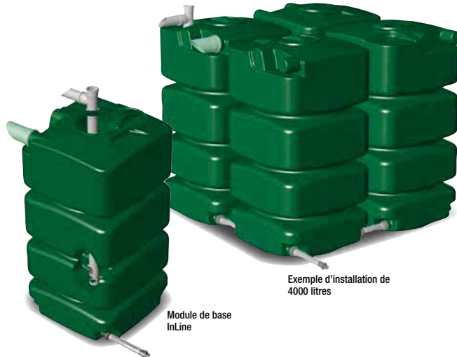
Réservoir InLine 800 - 78 x 78 x 156 cm - poids : env. 35 kg - module de base : JU3056 - module complémentaire : JU3057.
