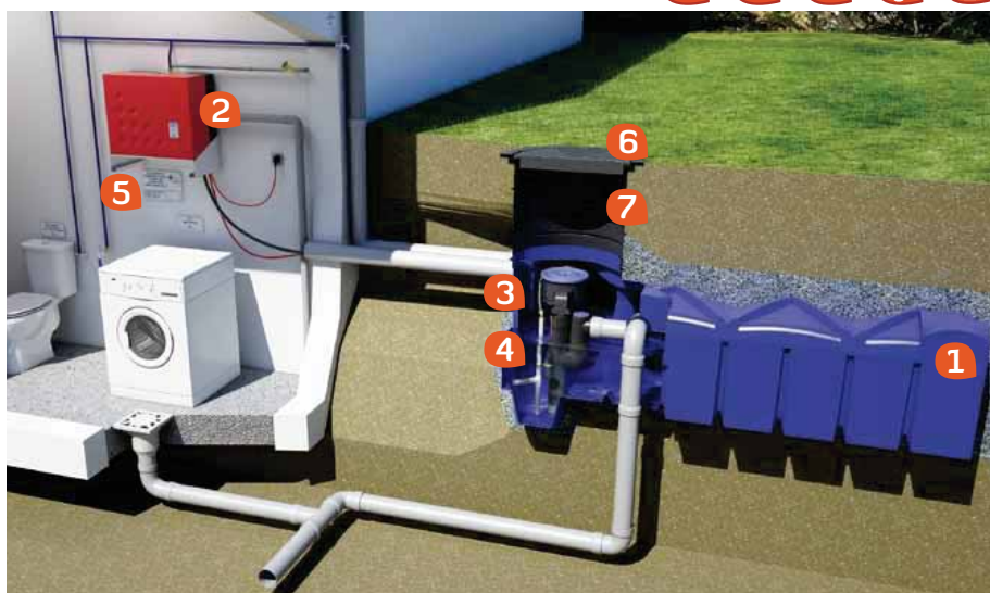
Exemple d'une installation de récupération d'eau de pluie composée de 2 F-Line 7500.
